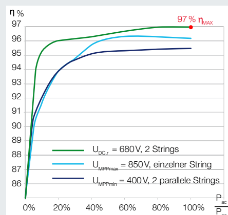
Wirkungsgradkennlinien PIKO 8.3
