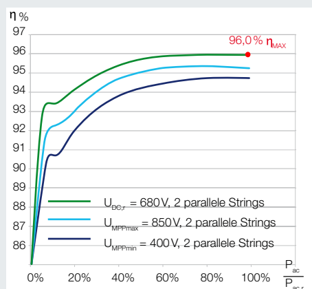
Wirkungsgradkennlinien PIKO 7.0
